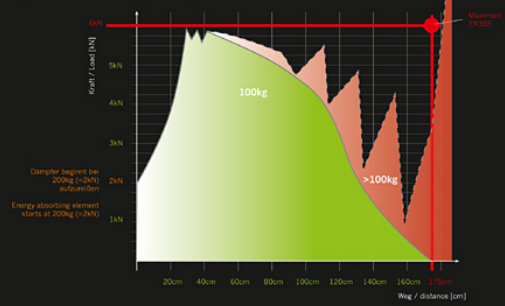
[DE] Kraft-Weg-Diagramm eines herkömmlichen Bandfedendämpfers [EN] Load-distance diagram of a usual textile energy absorbing element
