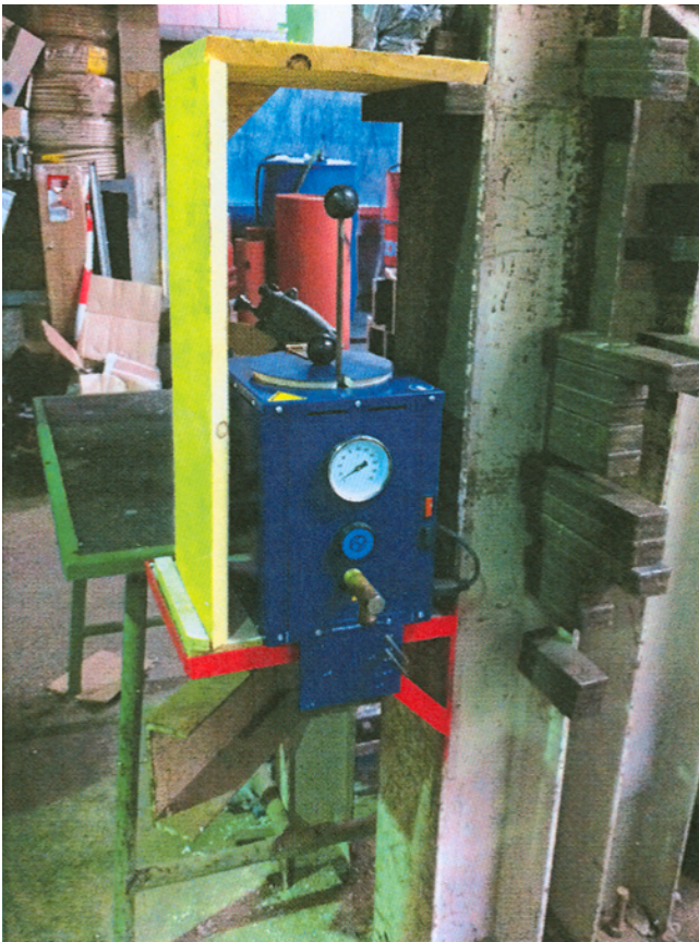
Vorschmelzer Außenschale
